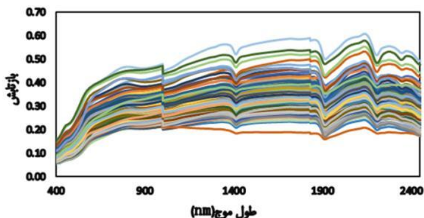
شکل ۲. میانگین منحنی‌های خام بازتاب
