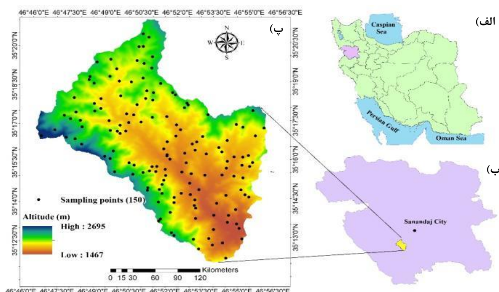
شکل ۱. موقعیت (الف) حوضه آبخیز کیلانه نسبت به کشور ایران (ب) در استان کردستان (پ) و توزیع مکانی نمونه‌های خاک: دایره‌های سیاه
