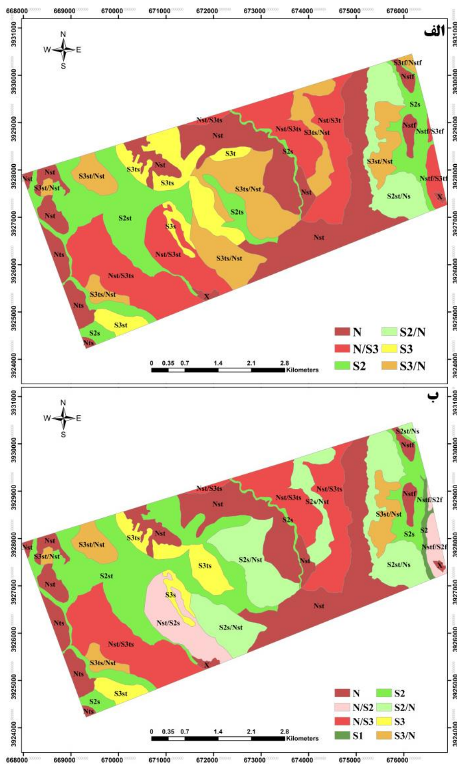
شکل ۴. کلاس‌های تناسب اراضی برای درخت بادام در شرایط فعلی (الف) و در شرایط آبی (ب)
