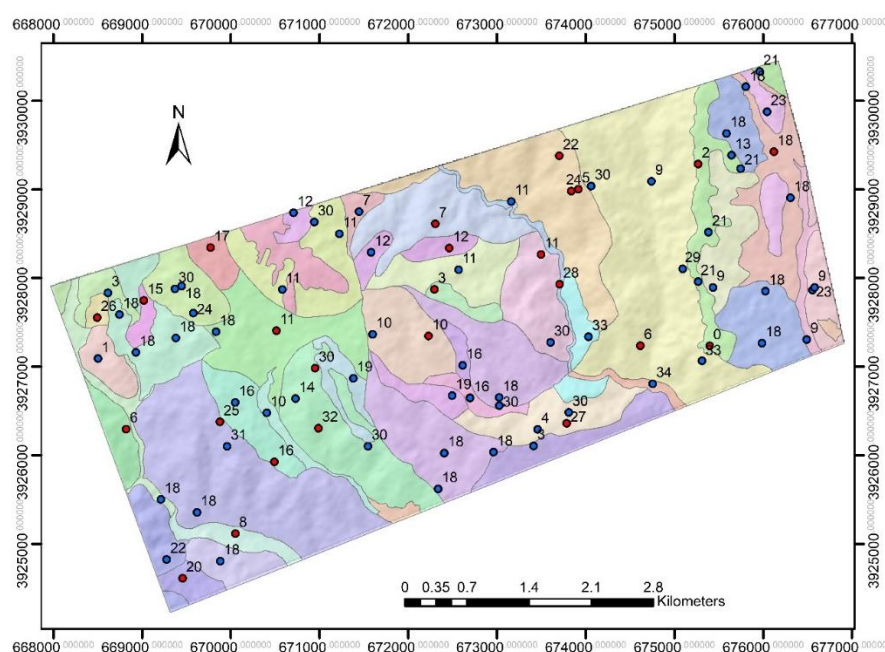
شکل ۲. نقشه خاک منطقه به همراه خاک‌رخ‌های حفر شده. خاک‌رخ‌های شاهد با رنگ قرمز مشخص شده است.
