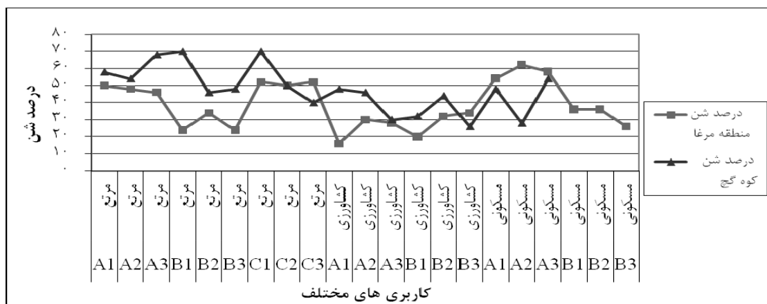
شکل ۵- ارزیابی درصد شن در کاربری‌های مختلف سازندهای گچساران و آغاچاری
