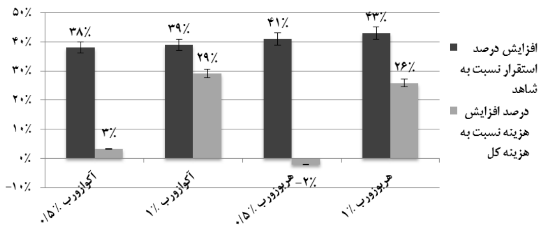
شکل ۵. میزان افزایش درصد استقرار و هزینه در واحد سطح با کاربرد فراچادب
