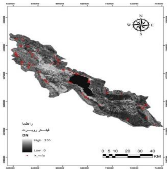
شکل ۱۳. فیلتر روبرت
