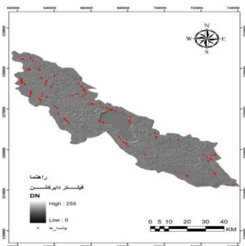
شکل ۱۱. فیلتر دایرکشن
