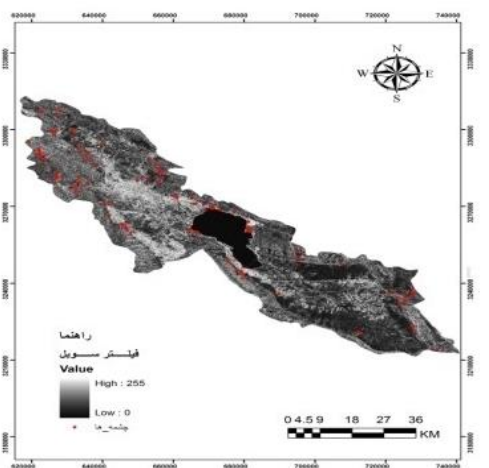
شکل ۱۲. فیلتر سوبل
