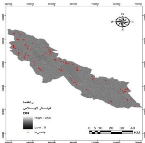
شکل ۱۰. فیلتر لاپلاس
