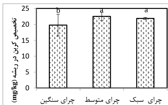
شکل ۶. نتایج مقایسه میانگین اثر شدت چرا بر مقدار تخصیص کربن در ریشه A. austriaca
