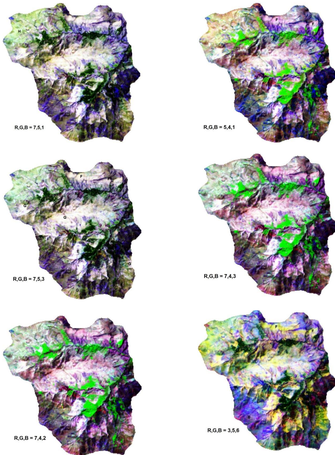
شکل ۲. نمونه‌هایی از ترکیبات رنگ مجازی (RGB) برای بارزسازی واحدهای سنگ‌شناسی
