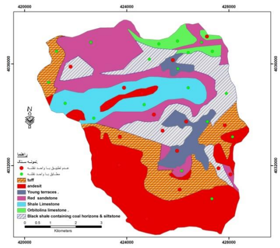
شکل ۳. نقشه زمین‌شناسی معمول به روش تفسیر عکس‌های هوایی، اقتباس شده از سازمان زمین‌شناسی
