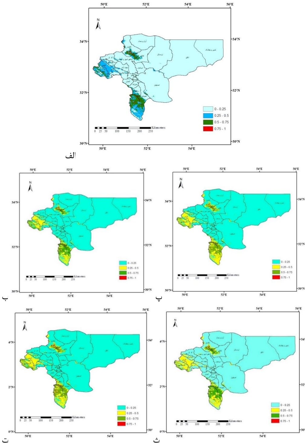
شکل ۴. نقشه‌های آشیان اکولوژیک اقلیمی حال حاضر و تحت سناریوهای اقلیمی سال‌های ۲۰۵۰ و ۲۰۷۰ گونه Br. Tomentellus در سطح استان اصفهان
