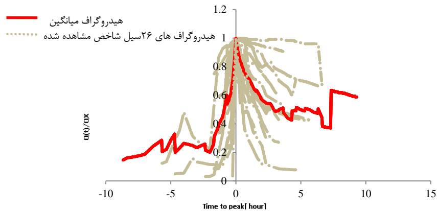
شکل ۶. هیدروگراف ۲۶ رویداد شاخص سیل و هیدروگراف میانگین آن‌ها در ایستگاه آب‌سنجی تنگ پنج بختیاری
