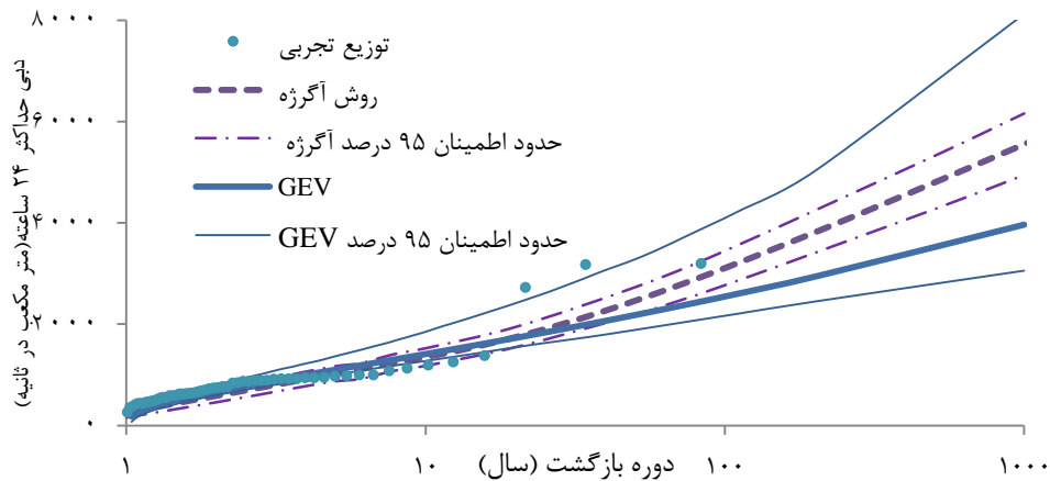
شکل ۳. برآورد روش‌های آگرزه و توزیع مقادیر حدی به همراه توزیع تجربی دبی‌های حداکثر ۲۴ ساعته در دوره بازگشت‌های مختلف و حدود اطمینان ۹۵ درصد هر یک از آن‌ها
