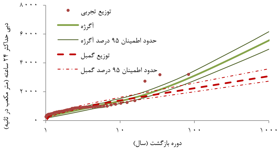
شکل ۴. برآورد روش‌های آگرژه و توزیع گمبل به همراه توزیع تجربی دبی‌های حداکثر ۲۴ ساعته در دوره بازگشت‌های مختلف و حدود اطمینان ۹۵ درصد هر یک از آن‌ها
